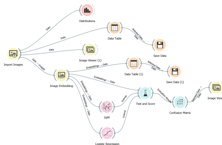
Gambar 5. Proses Klasifikasi
