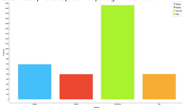
Gambar 2. Sebaran Dataset
